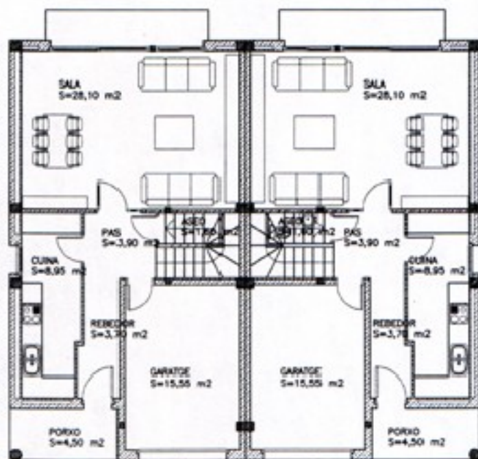
PLANTA BAIXA
