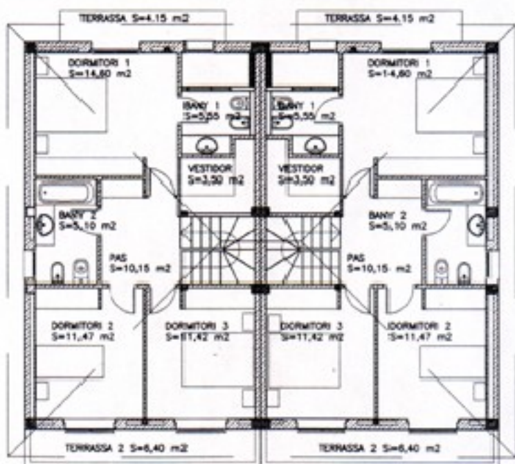
PLANTA PIS
